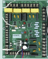
CZ-NS4P. PCB för avancerade funktioner så som 0-10V behovssignal, 2-zonskontrollfunktion, soldriven och extern switch
